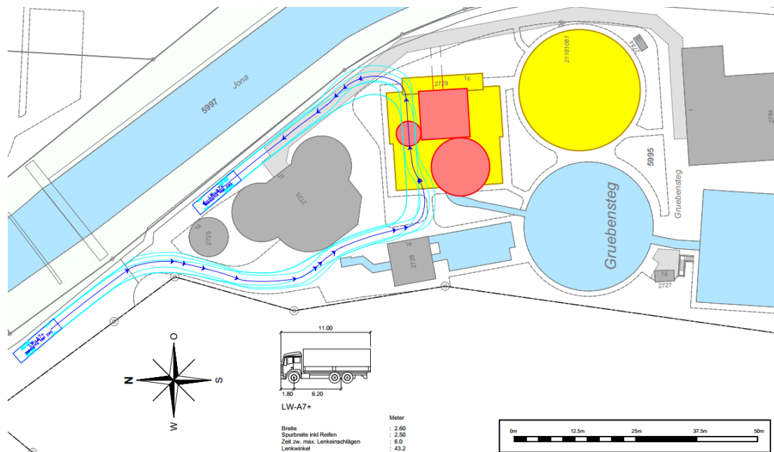
Abbildung 35: Schleppkurvenprofil für den Abtransport des entwässerten Schlammes
